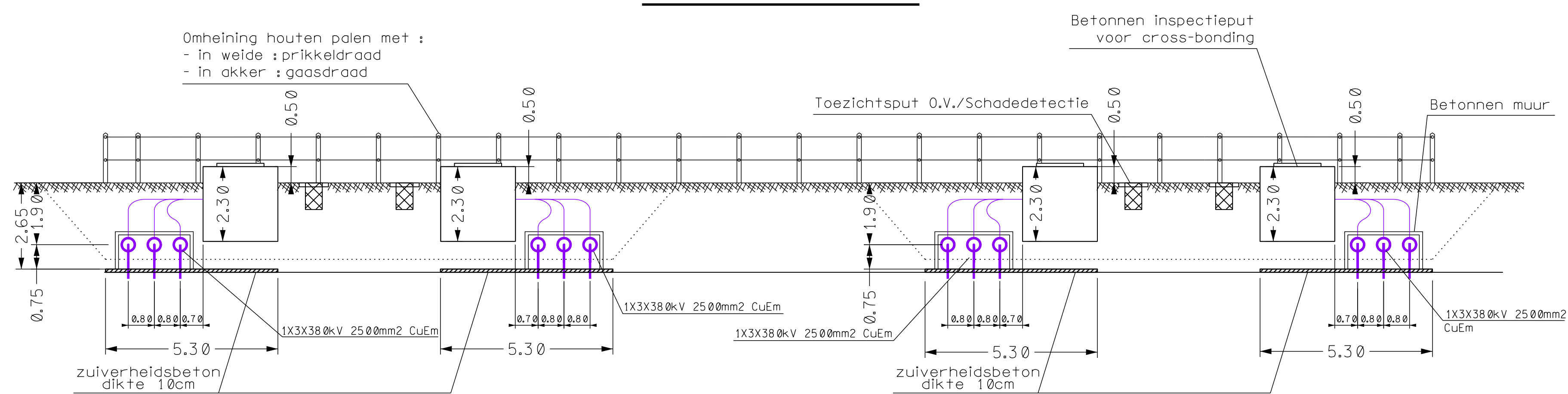
DWARSDOORSNEDE B-B'
